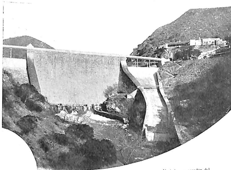
Vertedero y paredón del Dique San Roque, el mas grande depósito de irrigación de la Republica, admirable por si mismo y por su provecho real en favor de la riqueza agricola de la region.
